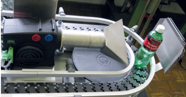
In Ablasanlage integrierter HOTWIND SYSTEM mit Breitschlitzdüse.
