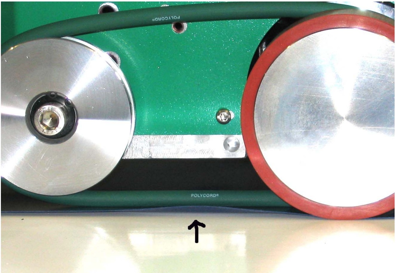
Oberliegende Folienkante zum leichteren Einführen der Schweissdüse anheben
